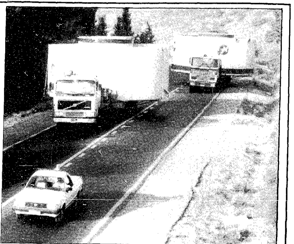
במסגרת פרויקט שימור איכות הסביבה, המתקיים במפעלים "דשנים" ו"חומרים מימיים" בחיפה, הועברו אתמול ארבעה מיכלים ענקיים, המיועדים לניטרול שפכים תעשייתיים, ממפעלי "נוימן" בנתניה לחיפה. כל מיכל מכיל 300 אלף ליטר, וקוטרו 8 מטר. במבצע העברת המיכלים, שארך בארבע שעות, השתתפו ארבע משאיות סמיטרילר. רוחבה של כל משאית - 8 מטר. בשל המבצע נסגרו לתנועה, עד תום ההובלה, כביש החוף וכביש ואדי-מילק. (כתב אריה קיזל, צילם רון סולומון)
